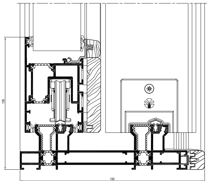
Sezione orizzontale
